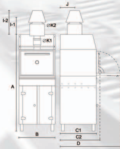
MEDIDAS HORNO-BRASA JOSPER MODELO L BC
